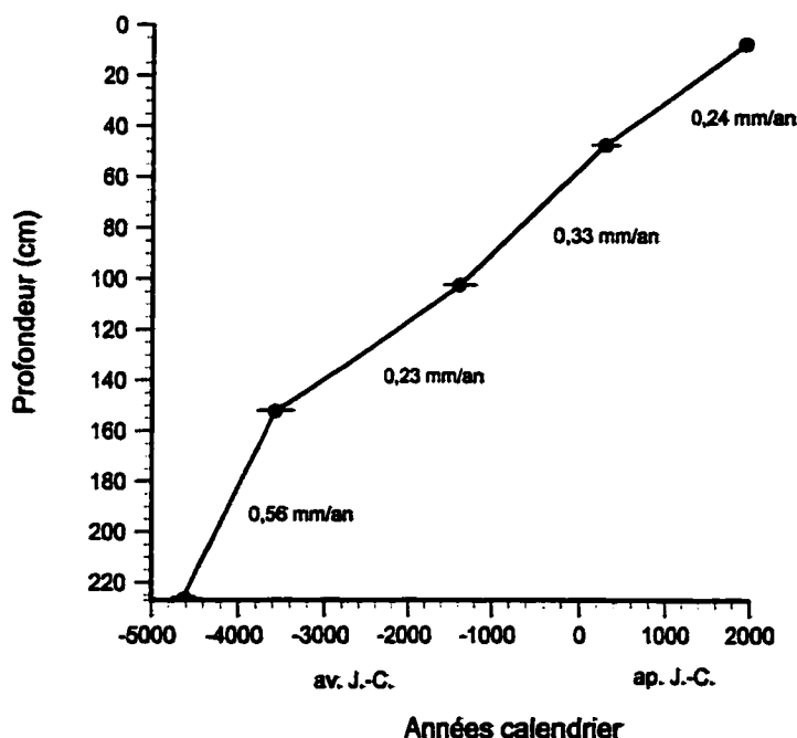
Fig. 3: Courbe d'accumulation de la tourbe (tourbière du mont du Lac des Cygnes).
