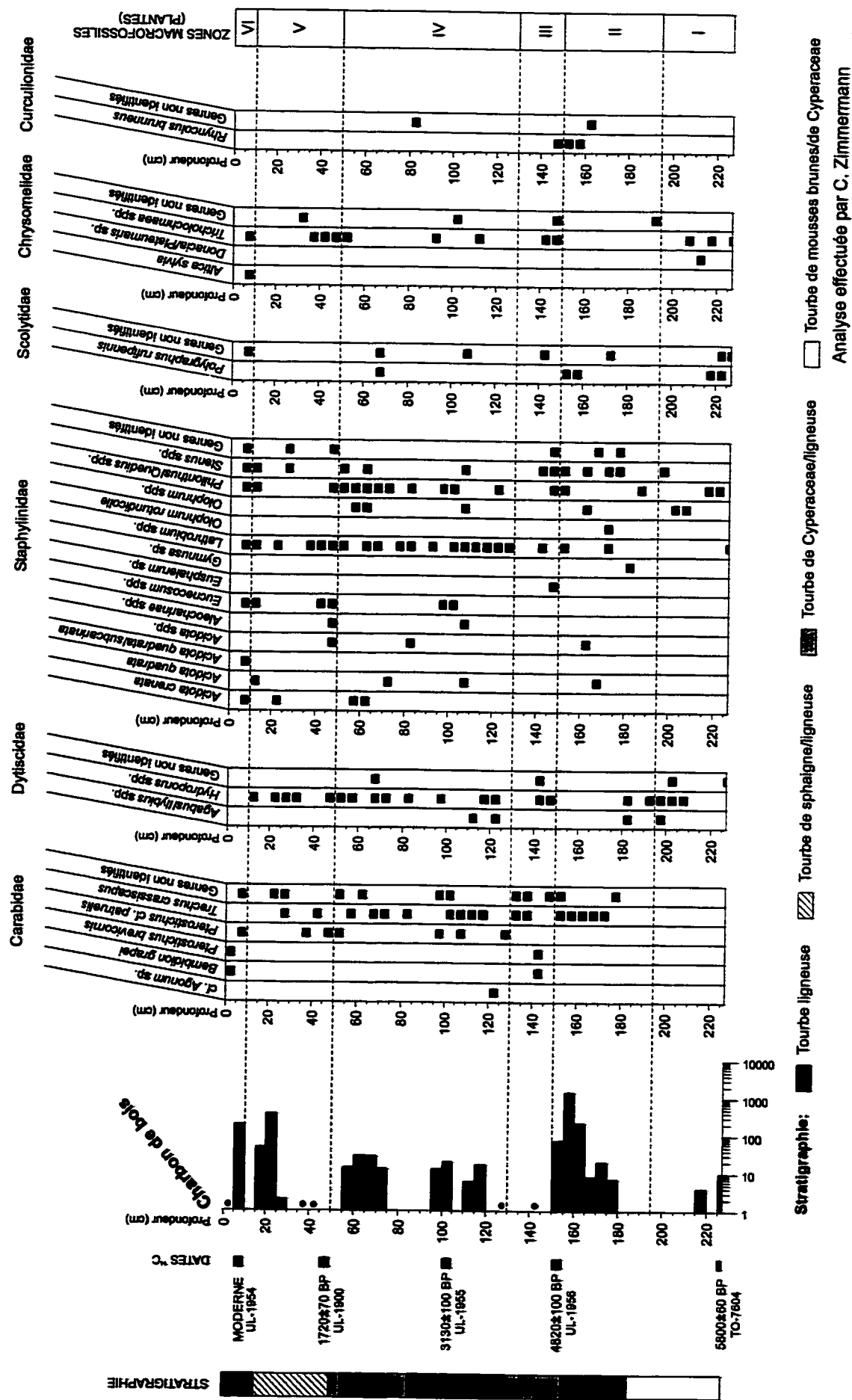
Fig. 6: Diagramme de présence des macrofossiles d'insectes (tourbière du mont du Lac des Cygnes, Charlevoix, Québec).
